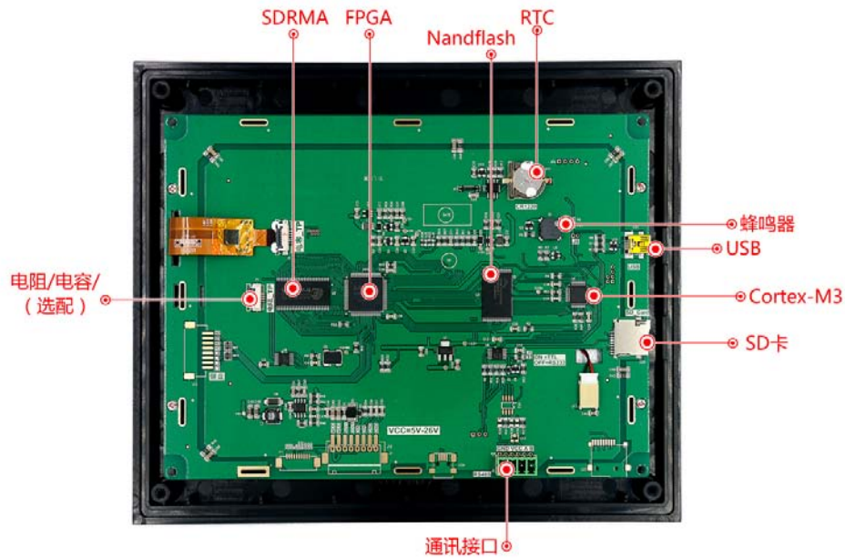
图 1-3 硬件配置图
